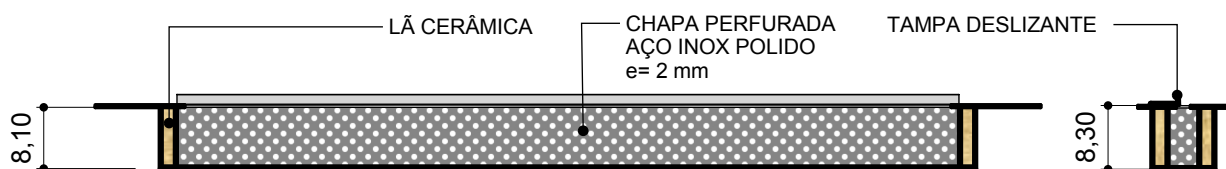
CORTES ESQUEMÁTICOS
